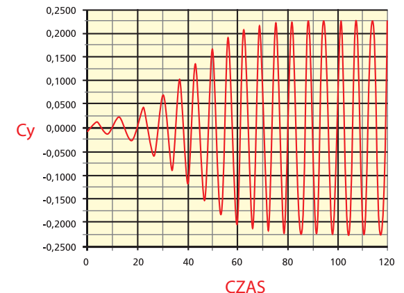
rys. 2. Wielkość drgań rury
